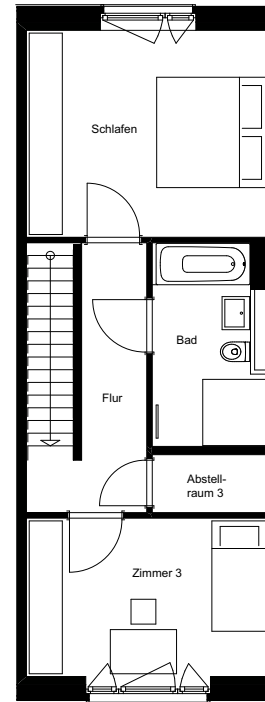
2. Obergeschoss
