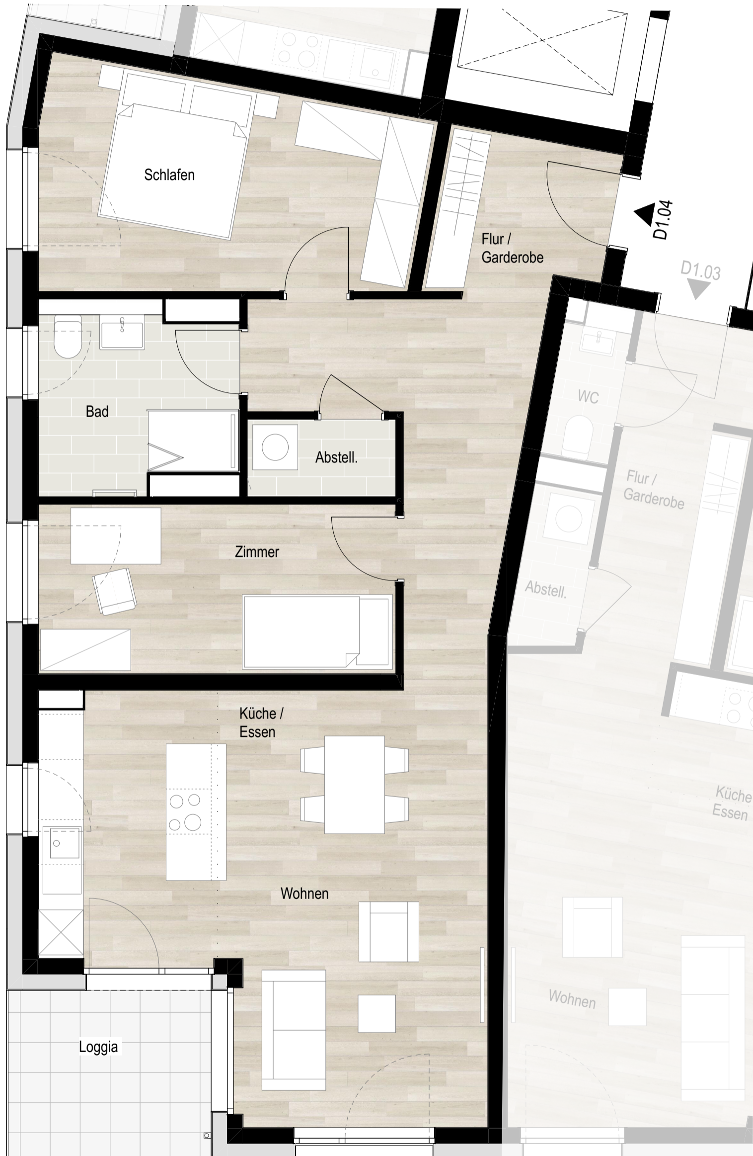
D1.04 1. Obergeschoss Süd-West
